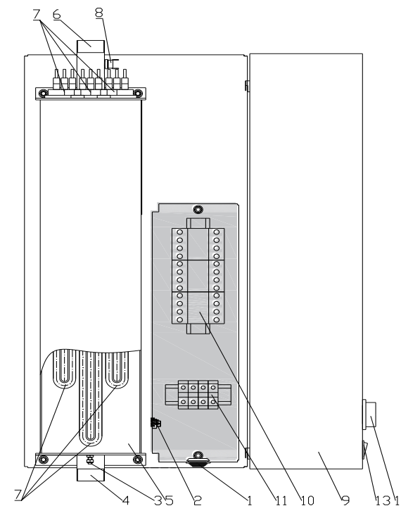
Рисунок 1. Устройство электрокотла. (крышка открыта)
