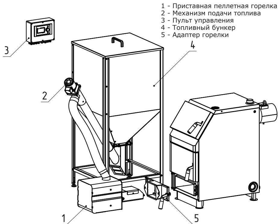
Рис. 1 Комплект приставной пеллетной горелки ZOTA Fox
