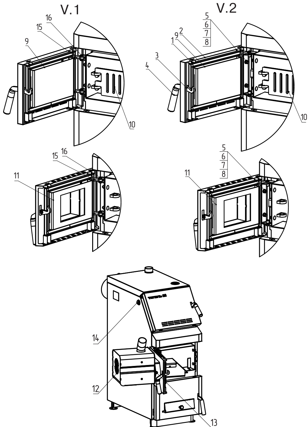
Рис. 12 Порядок установки адаптера на твердотопливные котлы ZOTA Тополь-М 42, 60, 80
