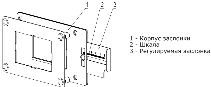
Рис.11 Заслонка вентилятора
