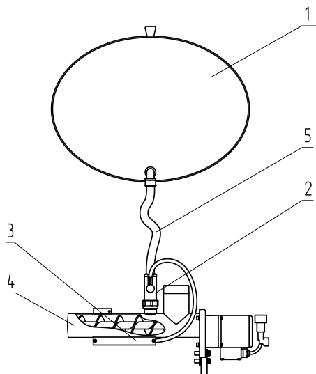
Рис.5 Система охлаждения топливопровода
